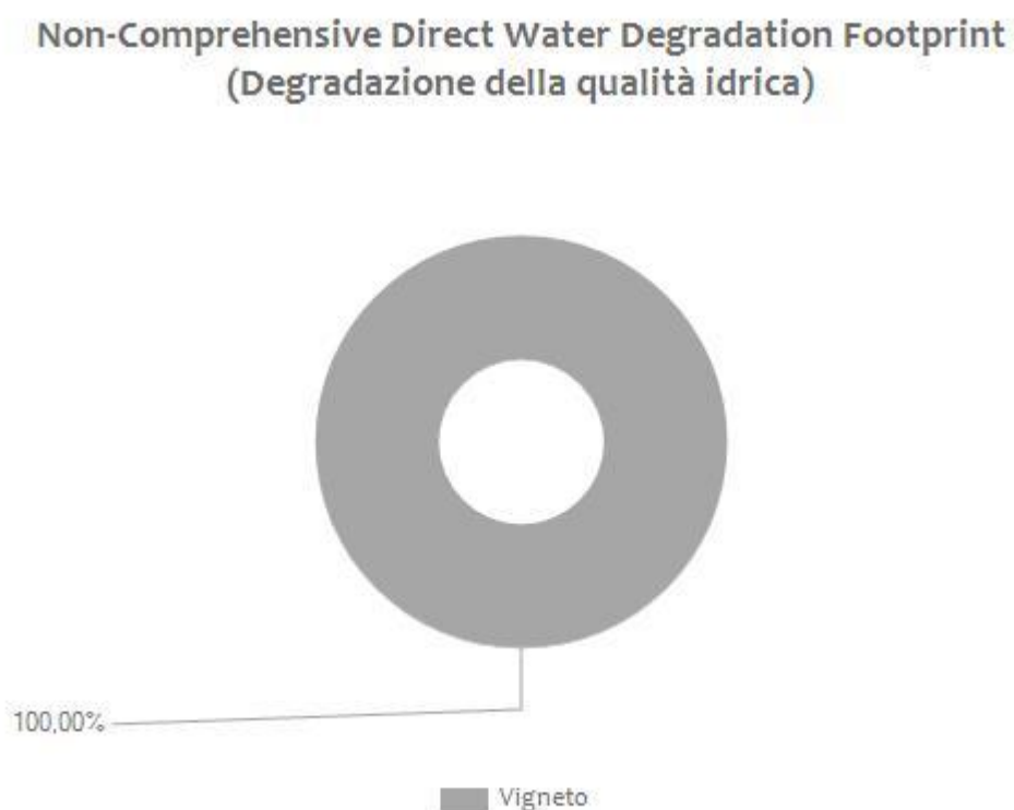
Figura 1 Valori percentuali dei diversi contributi rispetto a “Direct Water Scarcity Footprint” e “Non-Comprehensive Direct Water Degradation Footprint TOTALI” per l’azienda Soc. Agricola Tenute Rapitalà S.p.A.
