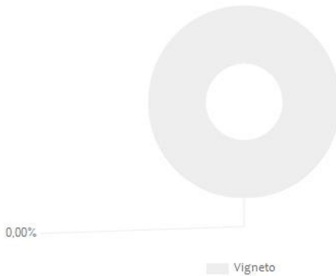
Figura 1. Valori percentuali dei diversi contributi rispetto a "Direct Water Scarcity Footprint" e "Non-Comprehensive Direct Water Degradation Footprint" TOTALI, per una bottiglia di Le Bacche Nere .
